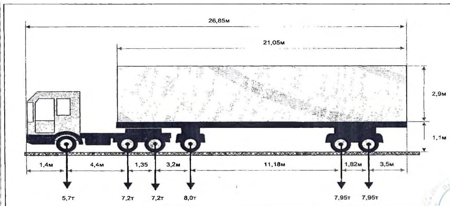
СХЕМА тяжеловесного и (или) крупногабаритного транспортного средства (автопоезда)
